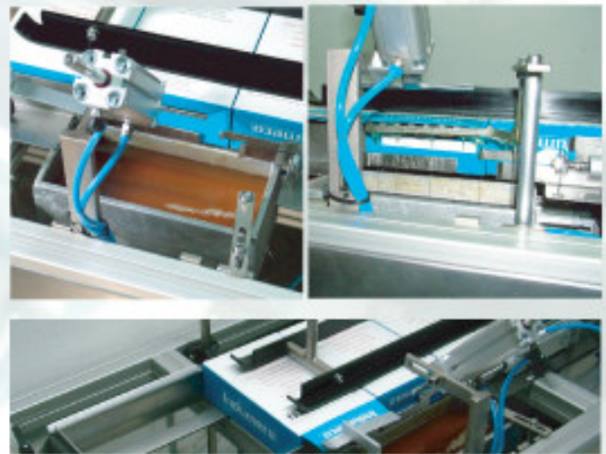
Encolado
